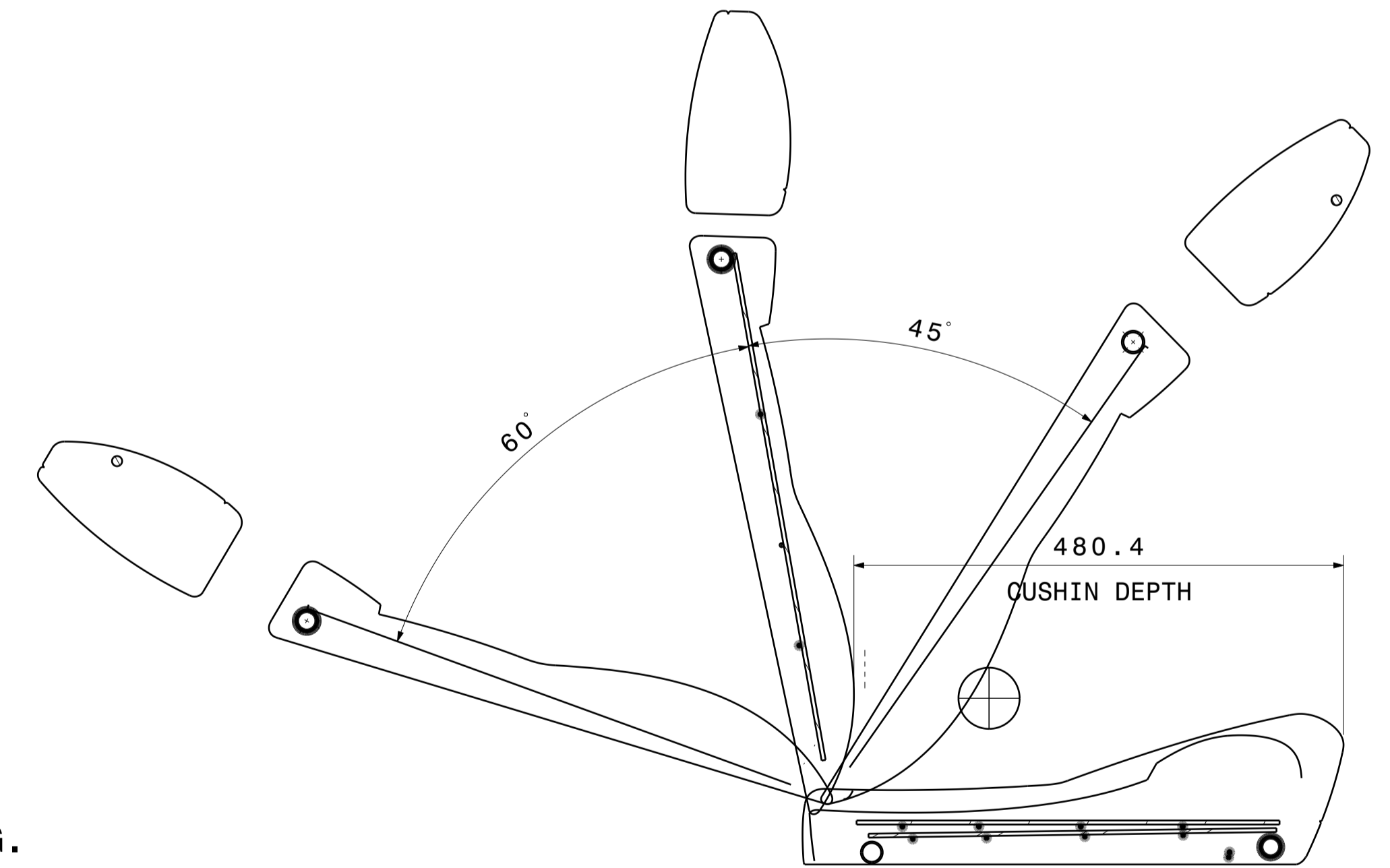
Section cut B-B Scale: 1:5
